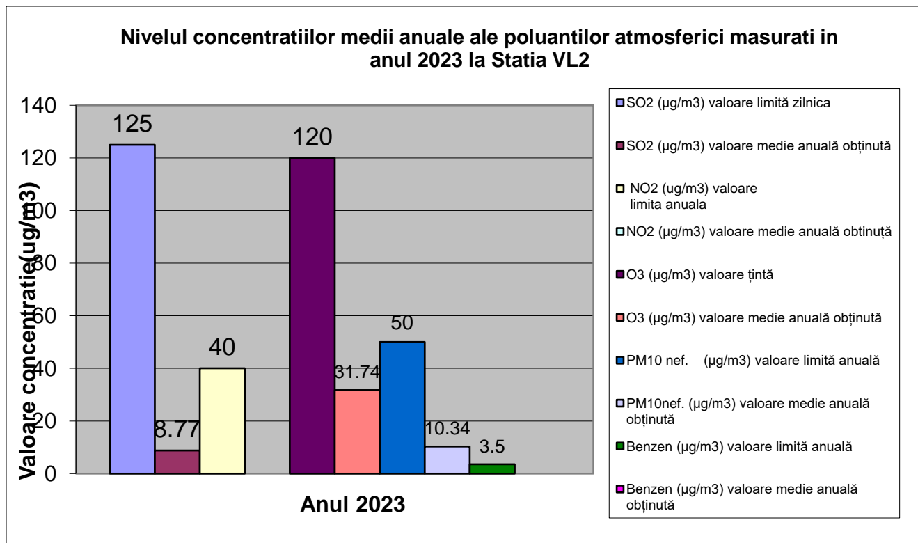
Graficul nr.2 Valorile indicatorilor monitorizați la nivelul județului Vâlcea la Stația automată de monitorizare a calității aerului VL 2 în anul 2023
