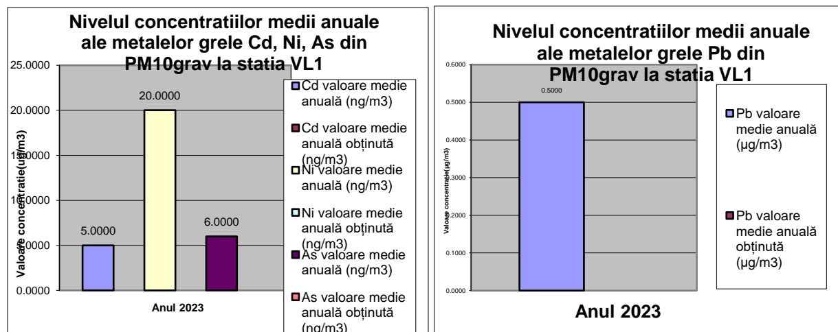
Graficul nr.4 Valorile medii anuale a concentrațiilor metalelor grele din fracțiunea PM10 grav. la Stația automată de monitorizare a calității aerului VL 1 la nivelul județului Vâlcea în anul 2023
