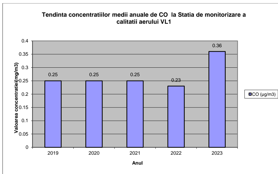
Graficul nr.3.2 Tendința concentrațiilor medii anuale ale CO monitorizat la nivelul județului Vâlcea la Stația automată de monitorizare a calității aerului VL 1 în perioada 2019-2023
