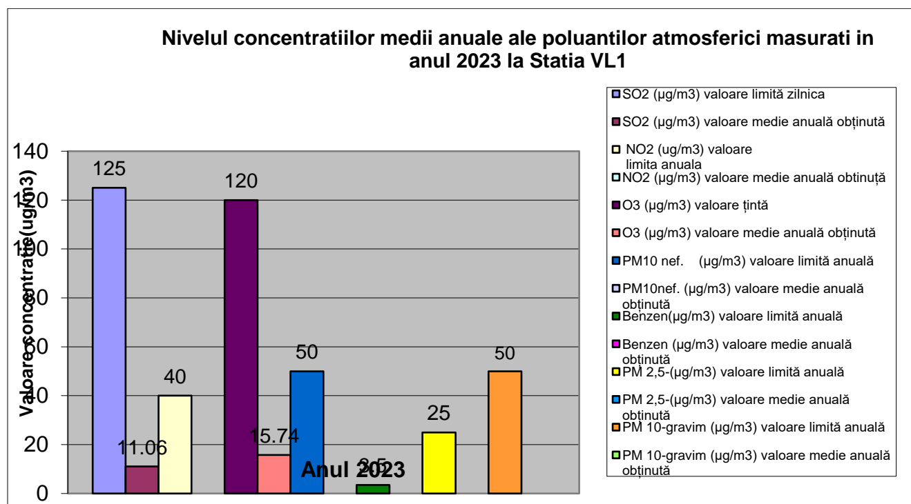
Graficul nr.1. Valorile indicatorilor monitorizați la nivelul județului Vâlcea la Stația automată de monitorizare a calității aerului VL 1 în anul 2023
