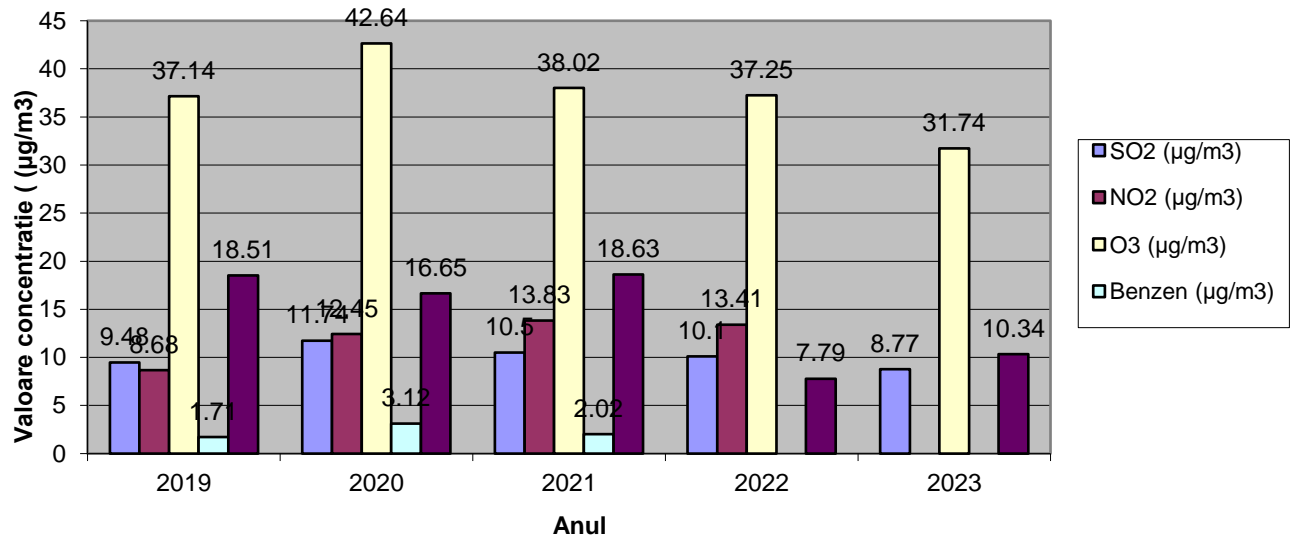
Graficul nr.3.3 Tendința concentrațiilor medii anuale ale poluanților atmosferici monitorizați la nivelul județului Vâlcea la Stația automată de monitorizare a calității aerului VL 2 în perioada 2019-2023
